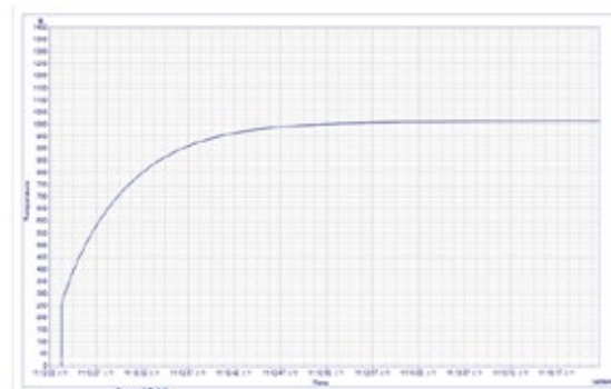
SN Heater Temperature( ^\circ\text{C} ).
